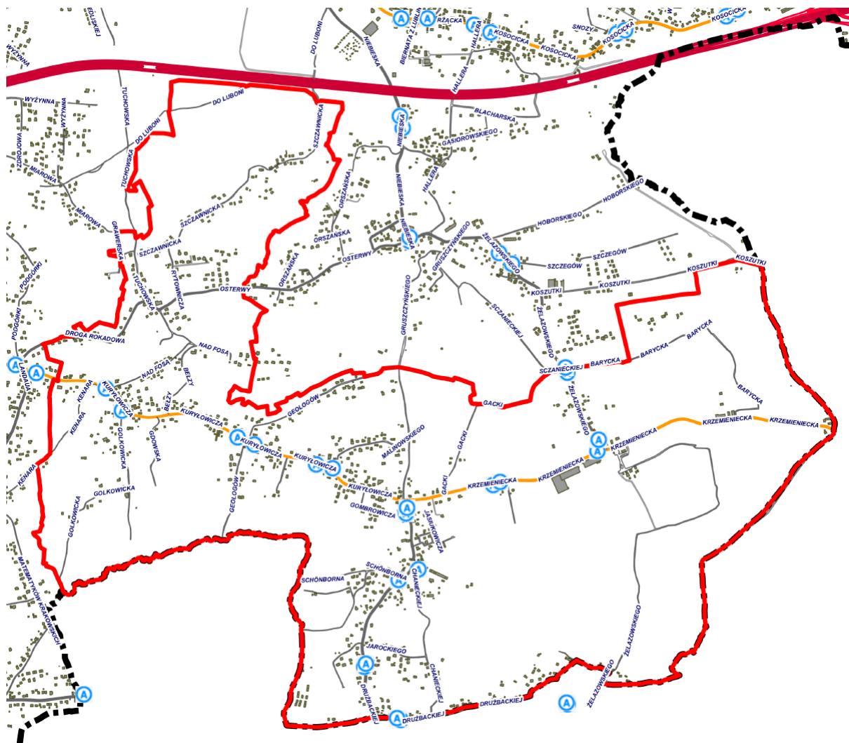
Rys. 3. Układ drogowy.
