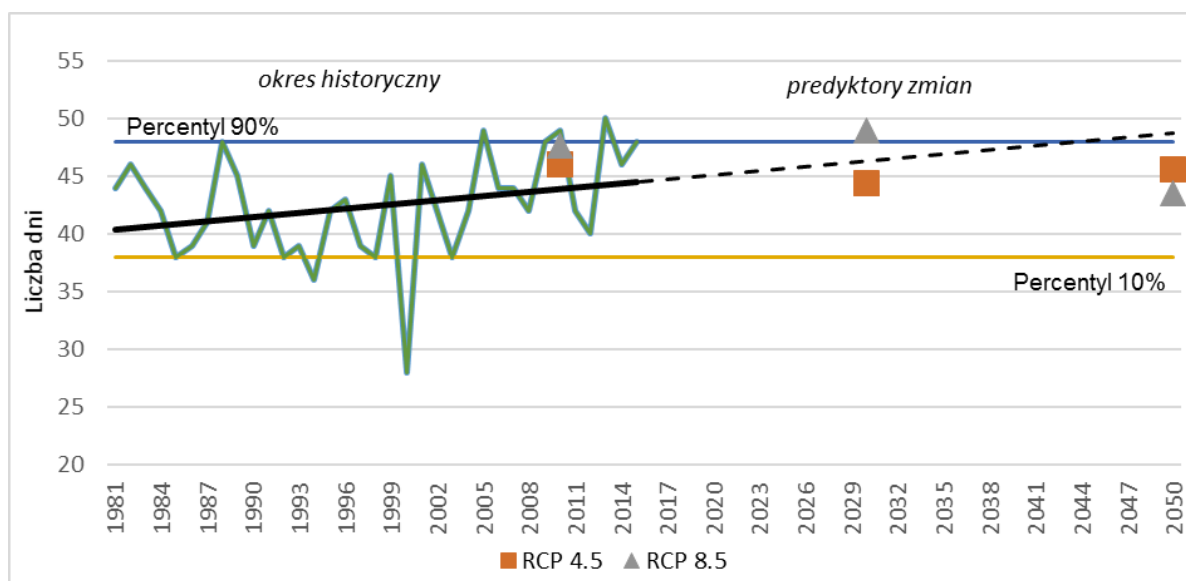
Rysunek 8. Liczba dni z opadem atmosferycznym przy temperaturze powietrza od -5 do 2,5^{\circ}\text{C}
