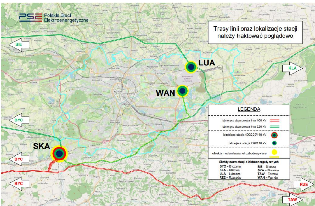
Rysunek 49 Schemat sieci przesyłowej na obszarze Gminy Miejskiej Kraków – plany na rok 2032.
