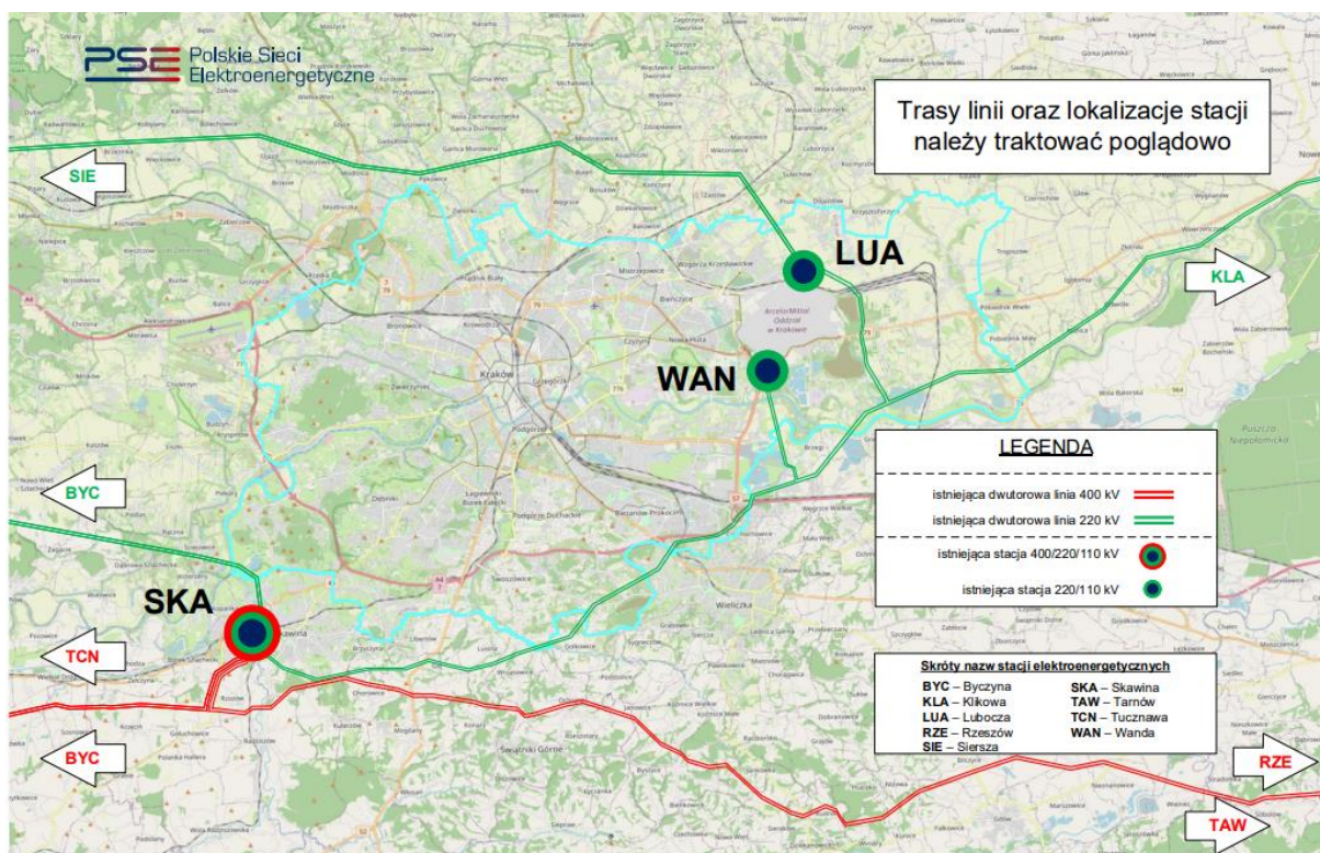
Rysunek 48 Schemat sieci przesyłowej na obszarze Gminy Miejskiej Kraków – stan istniejący.
