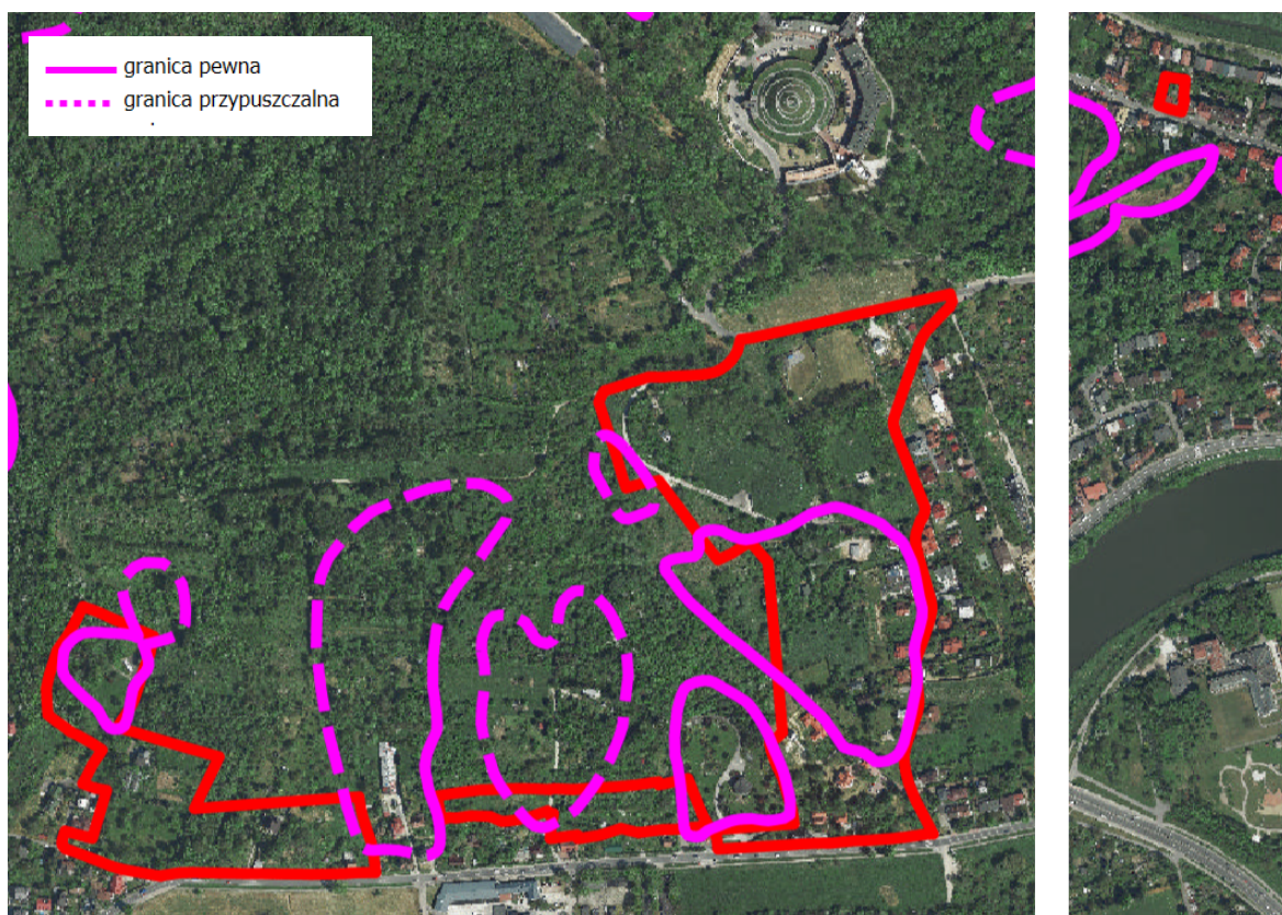
Rys. 7. Osuwiska w analizowanym obszarze
