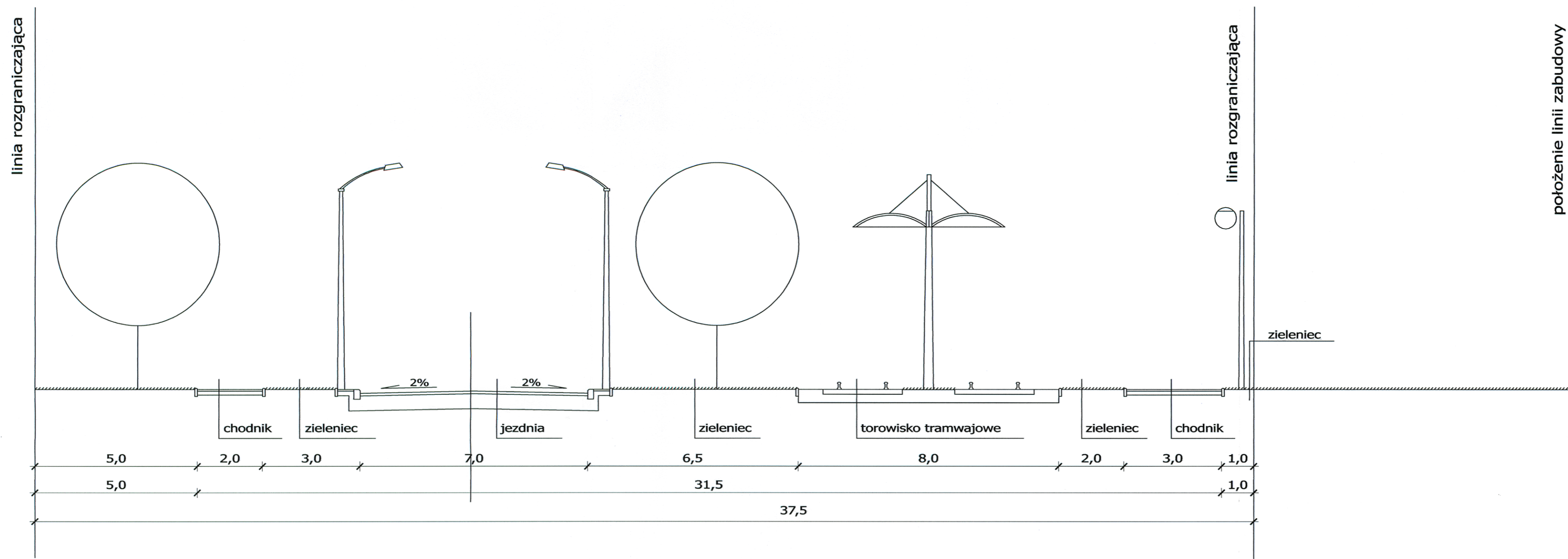
Przekrój typowy - ulica klasy KD/Z 1/2 + T
