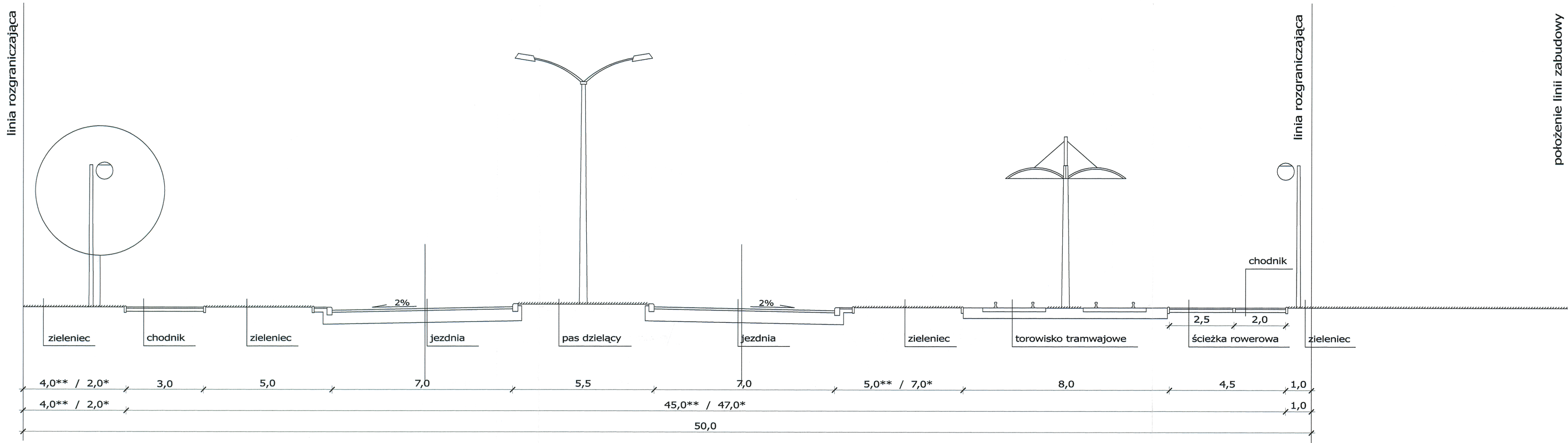
Przekrój typowy - ulica klasy KD/G 2/2+T (cz. północna)
