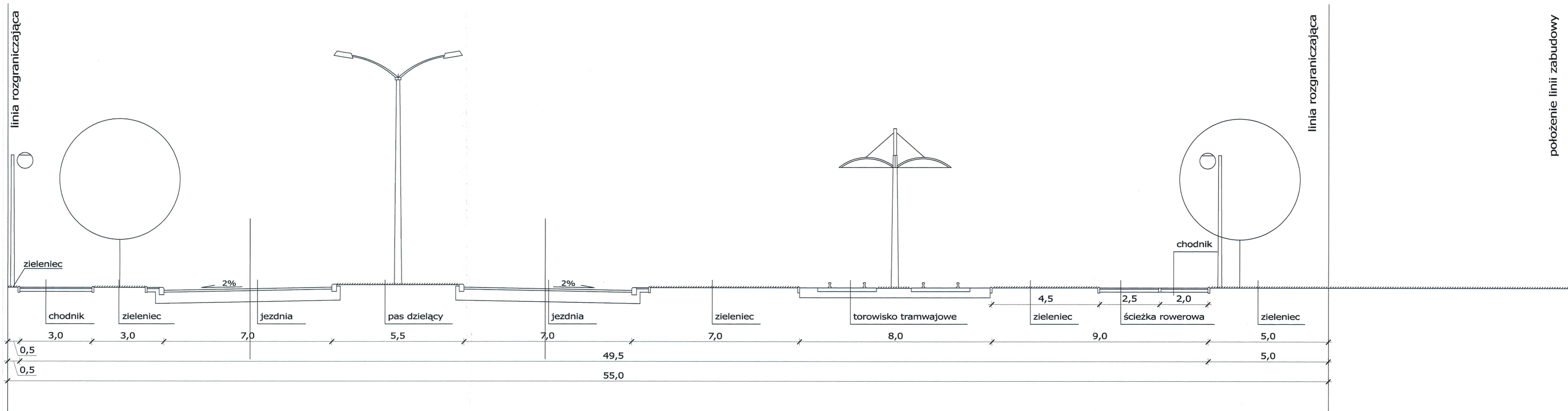
Przekrój typowy - ulica klasy KD/G 2/2 + T (cz. południowa)
