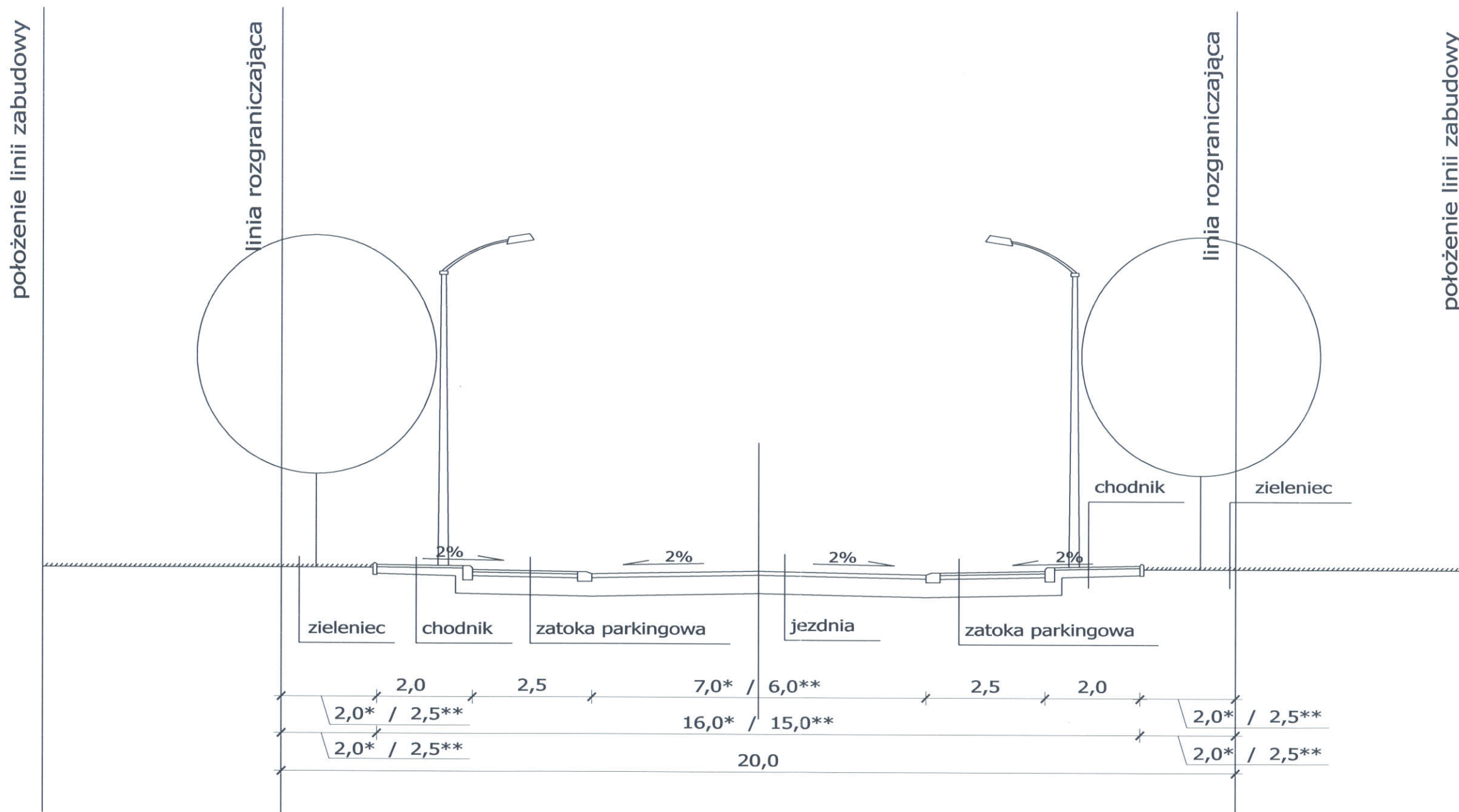
Przekrój typowy - ulica klasy KD/D (z obustronnymi zatokami parkingowymi)
