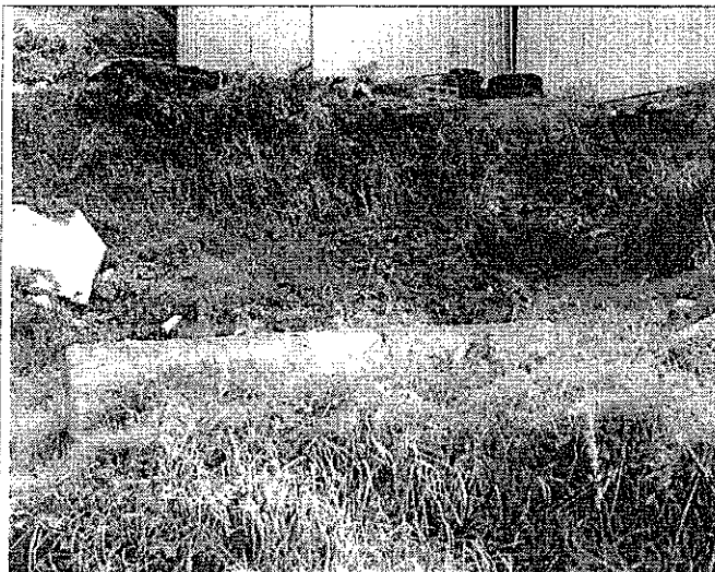
Skarpa główna osuwiska
