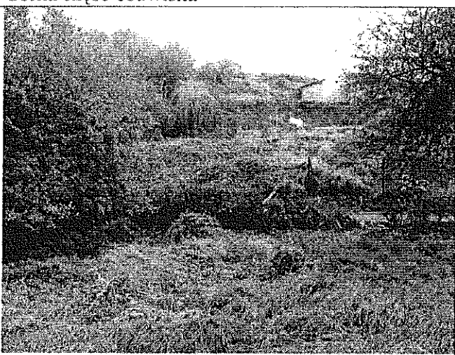
Czoło osuwiska, w górze skarpy głównej osuwiska
