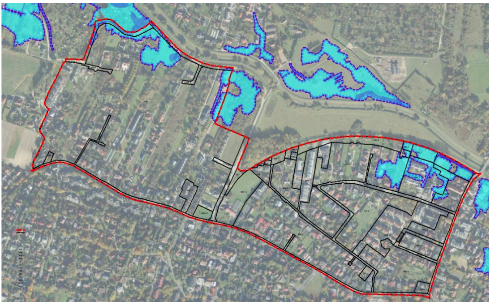
Ryc. 12. Obszar narażony na zalanie w przypadku całkowitego zniszczenia wału przeciwpowodziowego, przy wyznaczaniu którego przyjęto przepływ o prawdopodobieństwie wystąpienia 1% (raz na 100 lat) wg map zagrożenia powodziowego.
