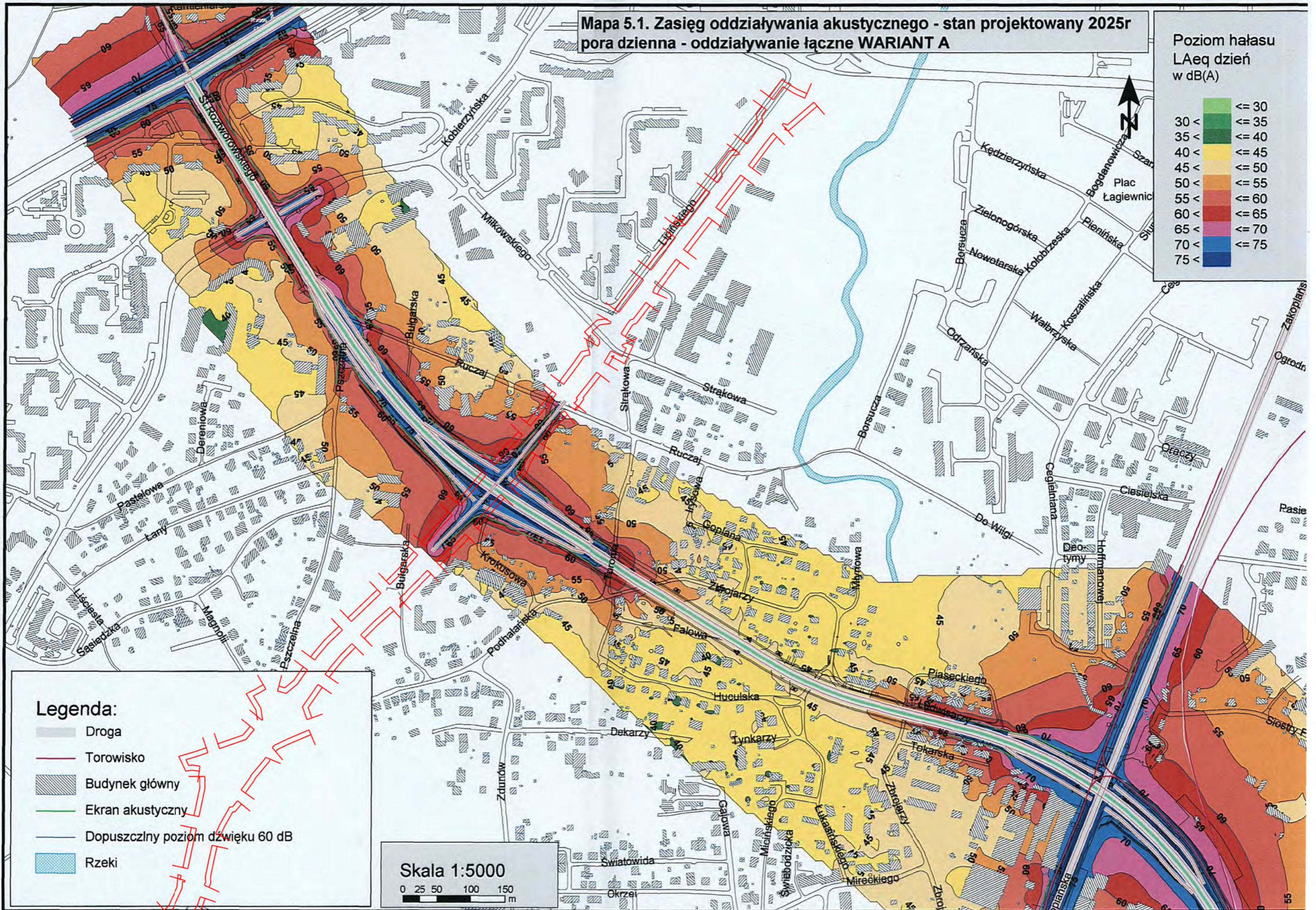
Zał.1. Zasięg oddziaływania akustycznego od projektowanej Trasy Łągiewnickiej - przebieg drogi w wariantcie z tunelem na odcinku pomiędzy ul. 8 Pułku Ułanów a ul. Zakopiąską
